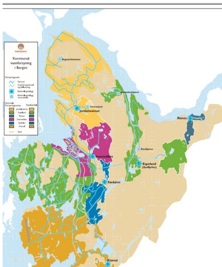
Figur 6 – Bergen vannforsyning 167
