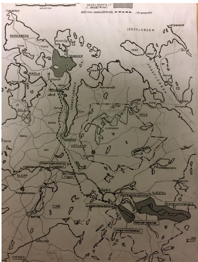
Figur 9 – Langevatn-utbyggingen 206
